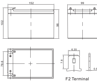
F2 Terminal
